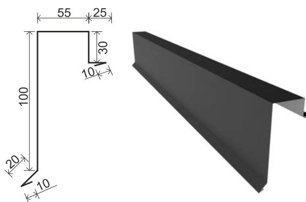
Планка з'єднання для фальцу 20/1 - 2м 80/1 - 0.48м
