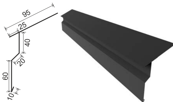
Вітрозахист для фальцу 5/1
