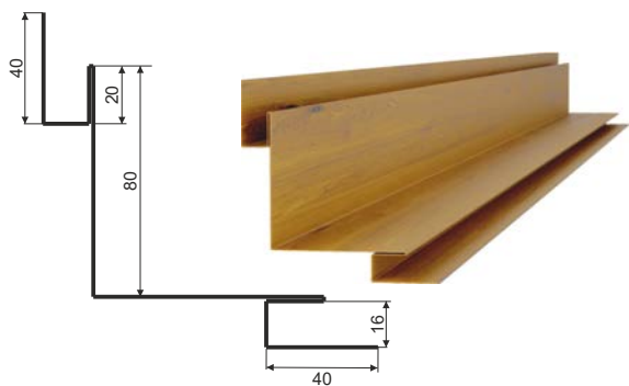
Кут внутрішній (тип 1) 4/1
