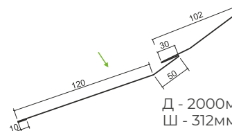
Планка перелому внутрішня 4/1
