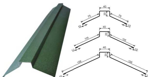
Декоративний 4/1
