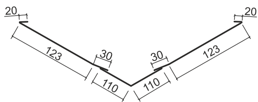
Жолоб плоский 2/1
