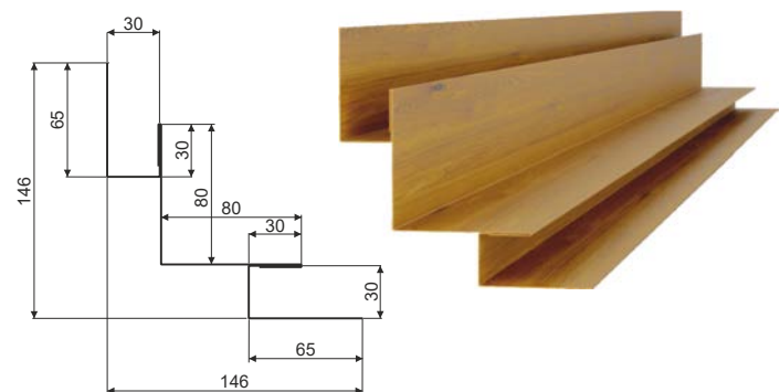
Кут внутрішній 2/1
