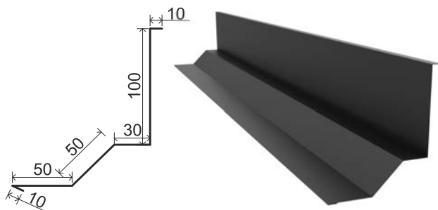
Стінний захист для фальцу 5/1
