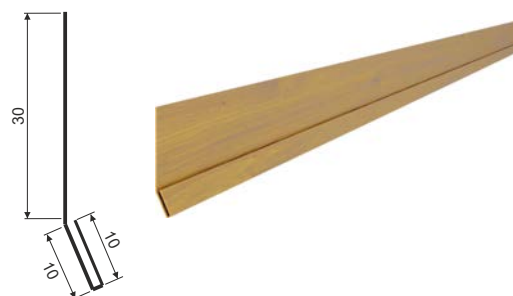
Планка стартова 25/1
