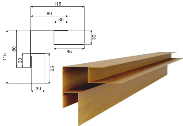
Кут зовнішній 2/1
