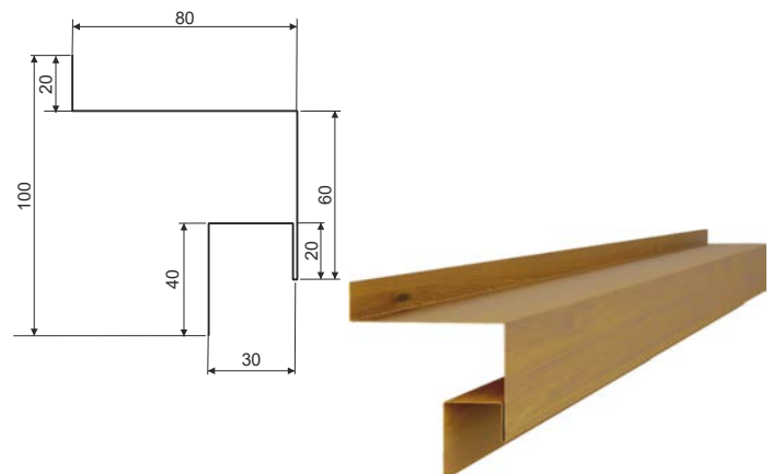
Зашивка підвіконника 5/1
