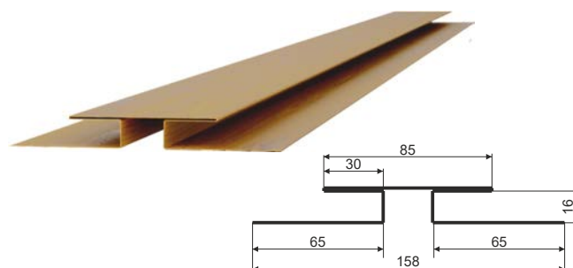
З'єднувальна планка 4/1
