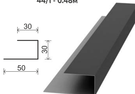
П-планка для фальцу 11/1 - 2м 44/1 - 0.48м
