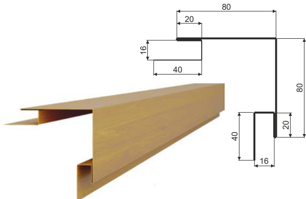
Зашивка підвіконника 5/1
