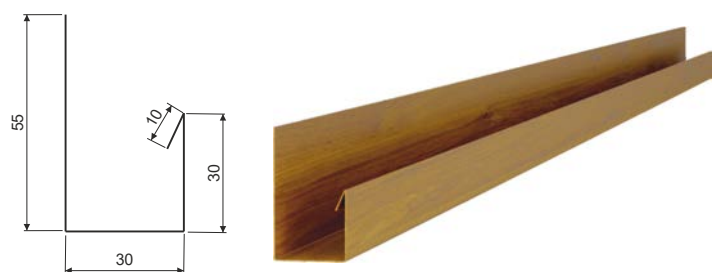
П-планка 10/1
