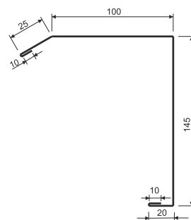
Для підшивки 4/1
