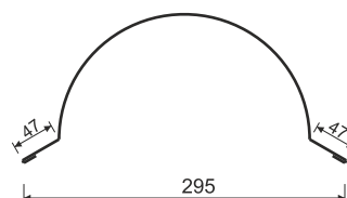
Заглушка конька велика
