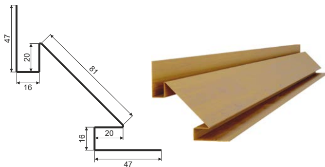
Кут внутрішній (тип 2) 5/1
