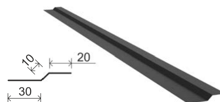
Планка з'єднання для фальцу 20/1 - 2м 80/1 - 0.48м
